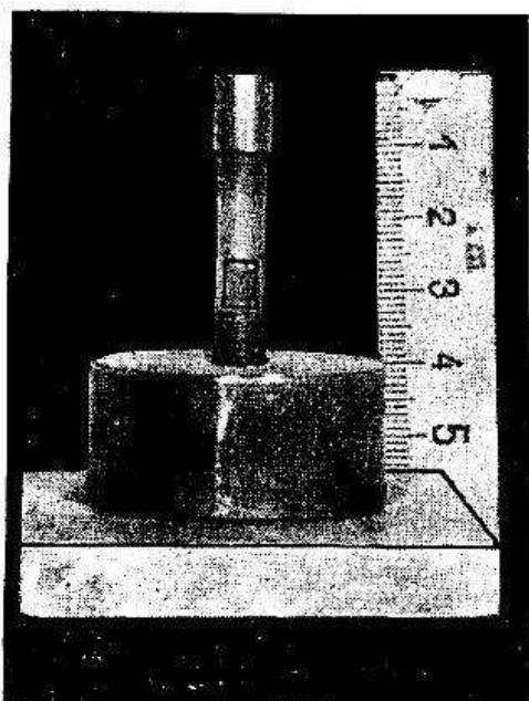
Obr. 3. Unikátne zariadenie vyvinuté v Ústave experimentálnej psychológie SAV inž. Vl. Valterom, umožňujúce registráciu nepozorovateľných pohybov. Jeho princíp tvorí magnetické teliesko so zrkadlom visiace na vlase, ktorý je pripevnený kvapkou oleja. Dosahuje sa tým zníženie odporu trenia na minimum, čo umožňuje registráciu aj takých mikropohybov, akými sú napr. priebeh a zánik nepozorovateľných pohybov po klinickej smrti organizmu.
